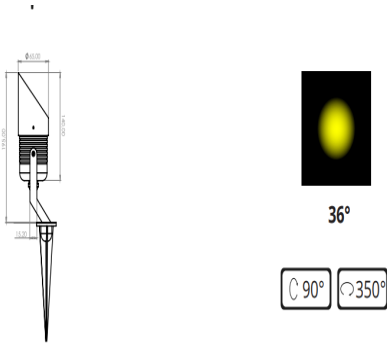
Teknik Çizim ve Işık Dağılımı
