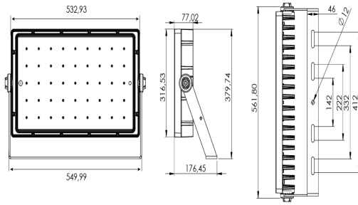
Teknik Çizim
