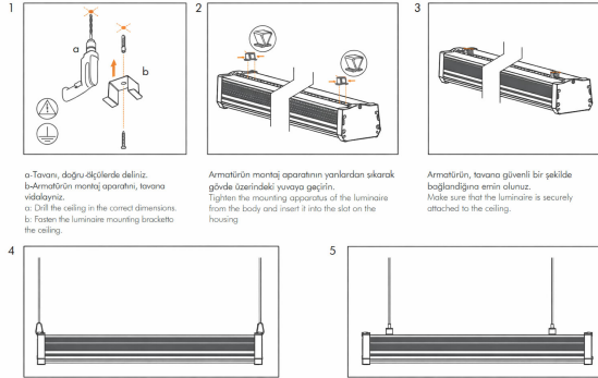
Montaj Detay
