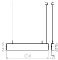
LINEA Svaüstü Teknik Çizim ve Ilık Açsı
