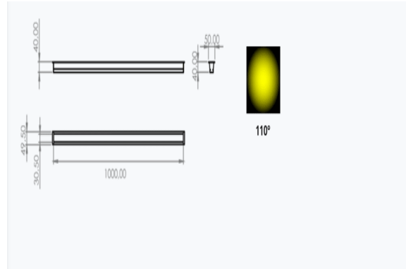
LINEA Svaalt Armatür Teknik Çizim
