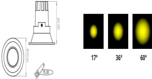
Teknik Çizim ve Işık Dağılım Grafiği
