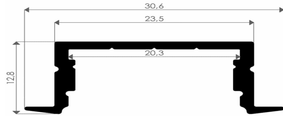
Siyahı Ledbar Teknik Çizim
