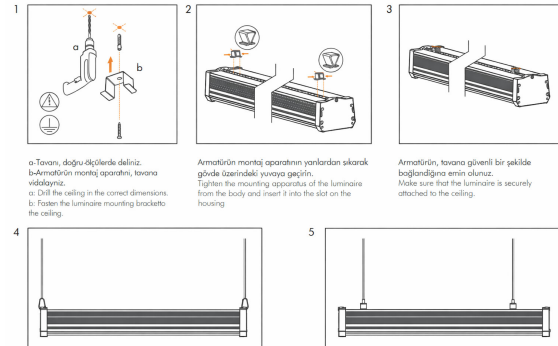
Teknik Çizim
