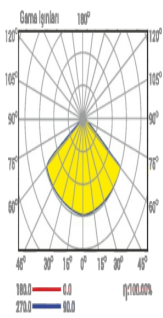
Spektrofotometrik Ölçüm
