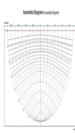
Isocandela Diyagramı
