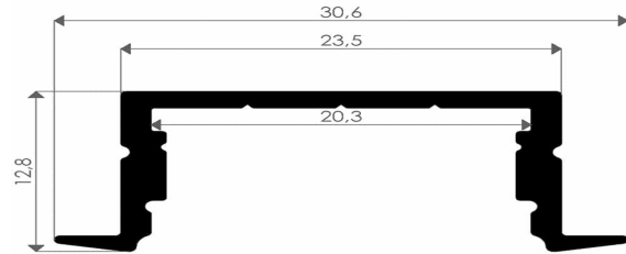
Sivaaltı Ledbar Teknik Çizim
