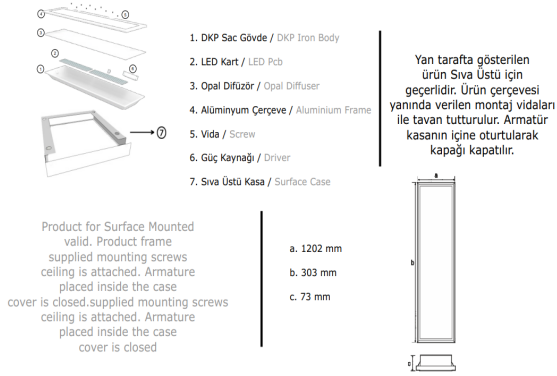
Teknik Çizim & Montaj
