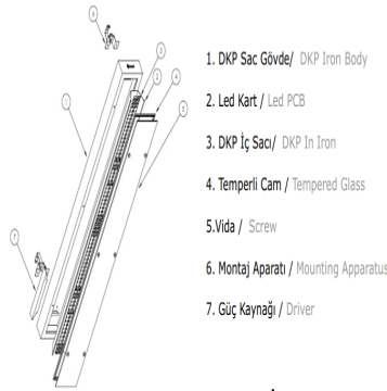
Teknik Çizim
