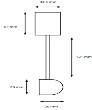
Montaj Ölçüleri
