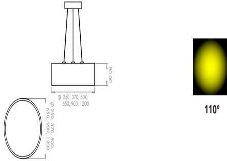
Teknik Çizim ve Işık Dağılımı
