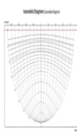
Isocandela Diyagramı
