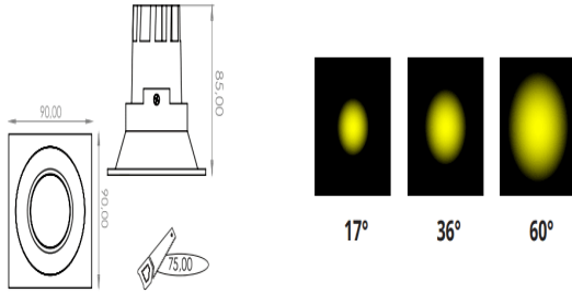
Teknik Çizim ve Işık Dağılımı
