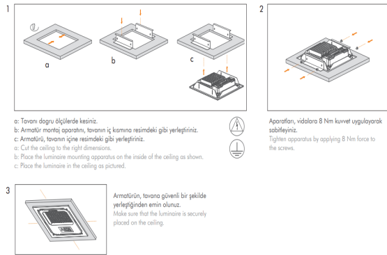
Montaj Detay
