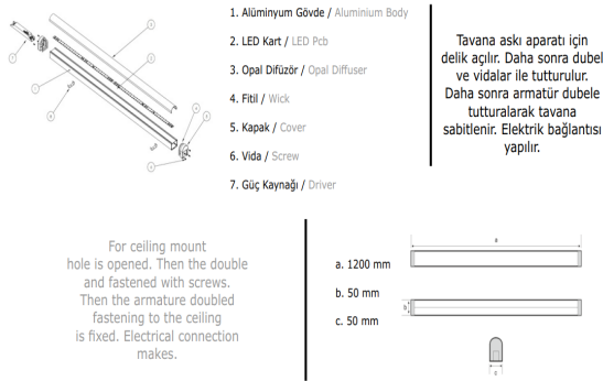
Teknik Çizim ve Boyutlar
