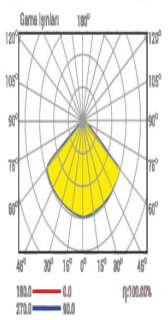
Spektrofotometrik Ölçüm
