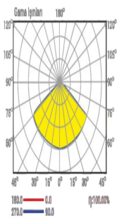
Spektrofotometrik Ölçüm
