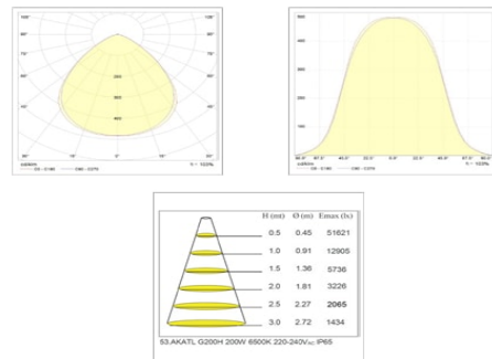
Fotometrik Veriler
