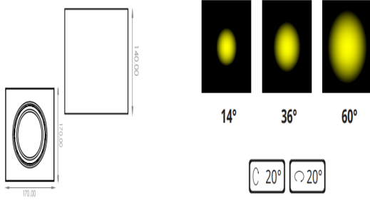
Teknik Çizim ve Işık Dağılım Grafiği
