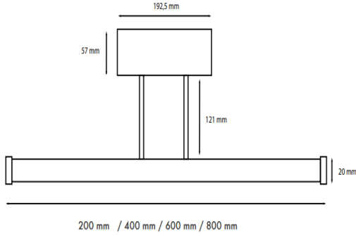
Teknik Çizim
