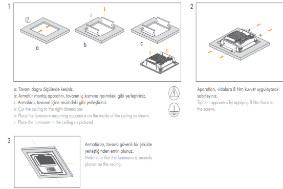
Montaj Detay
