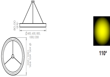
Teknik Çizim ve Işık Dağılımı
