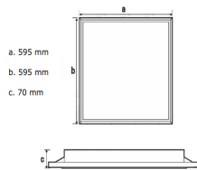
Montaj Detay
