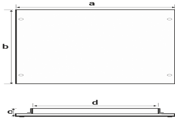
Teknik Çizim
