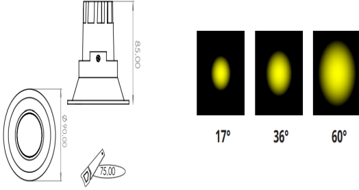
Teknik Çizim ve Işık Dağılımı
